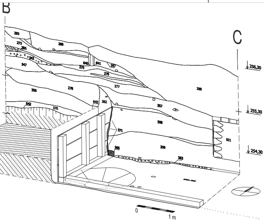
obr. 5 Opava, Pekařská ulice č. o. 13, výzkum 2002. Perspektivní pohled na profil souvrstvím se sutérénem k. 643 s pokusem o rekonstrukci podoby jeho vnitřní dřevěné konstrukce.
