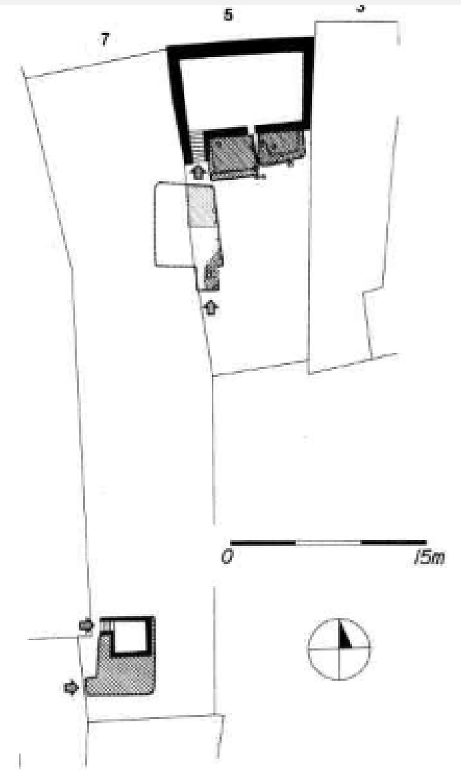
Obr. 3: Brno, Velký špalíček, Dominikánská 5 a 7, půdorys parcel v úrovni suterénu s vyznačením dřevohliněné a kamenné zástavby ze 13. století. Černě kamenná jádra, šrafovaně dřevohliněné suterény.
