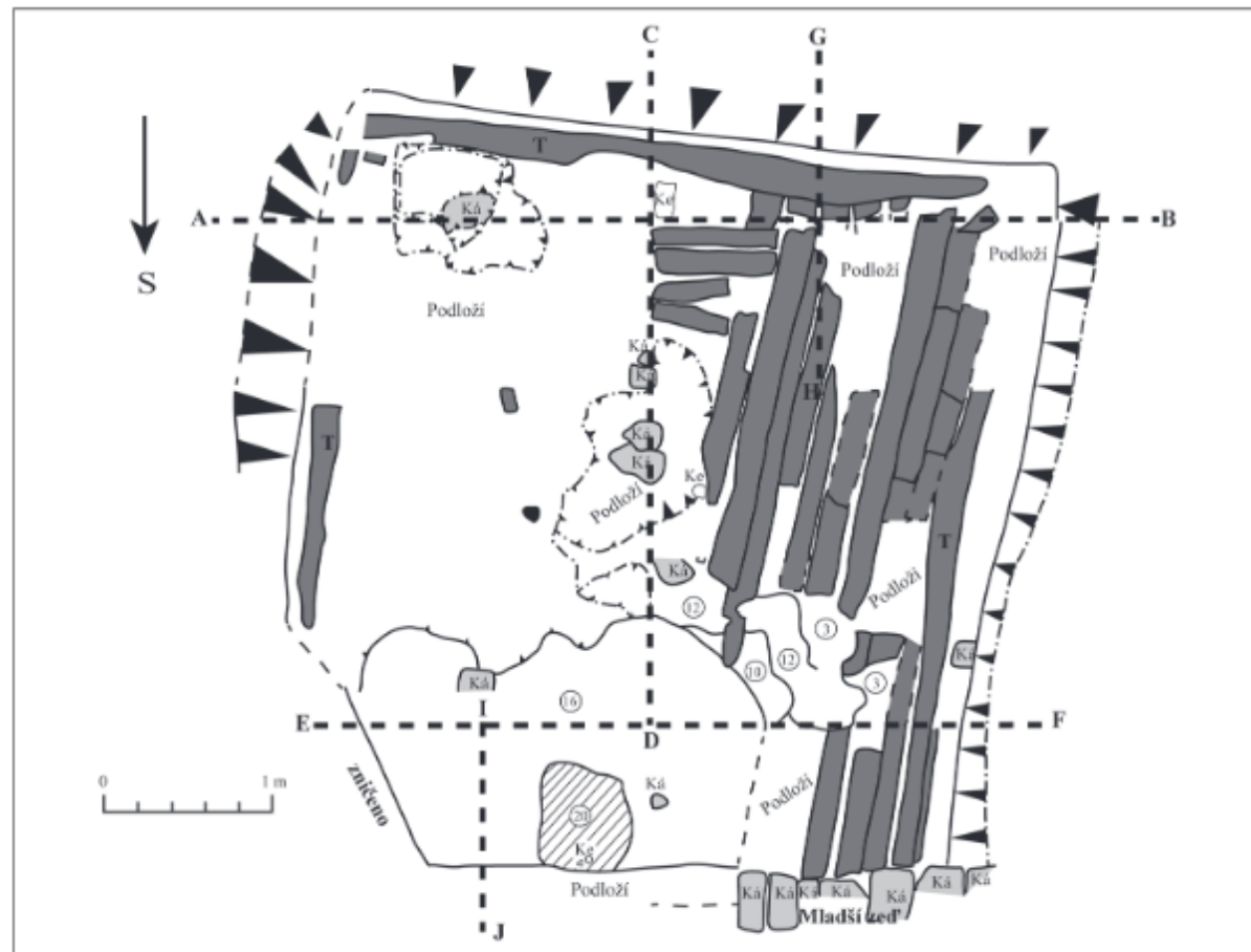
Obr. 3. Půdorys zahloubeného objektu. Tmavě šedě – dřeva (T = trámy, ostatní jsou prkna a jiná dřeva), světle šedě – kameny, čarofáním vyznačeno místo ohniště. V kružnicích čísla vrstev.
