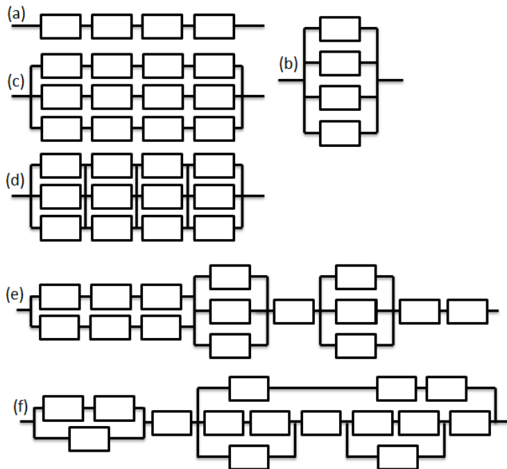
Obrázek 7.2: Příklady řazení výrobních linek: (a) čistě sériové řazení, (b) čistě paralelní řazení, (c) paralelně-sériové řazení bez křížení, (d) paralelně-sériové řazení s křížením (e) hybridní řazení, (f) multiprocesní řazení
